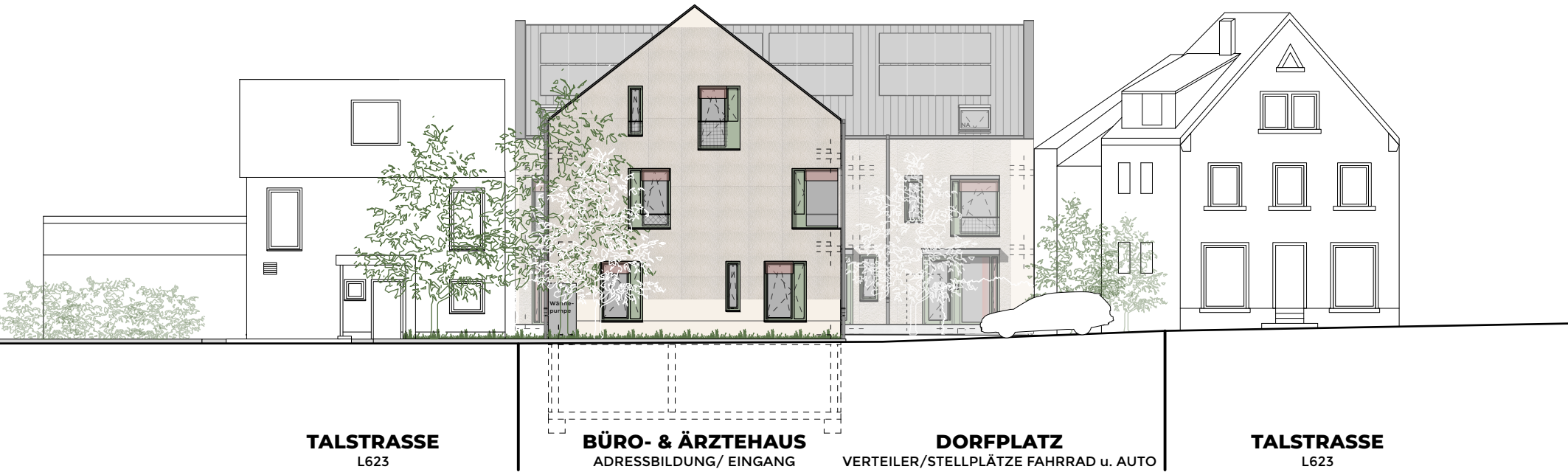
Ansicht Talstrasse
