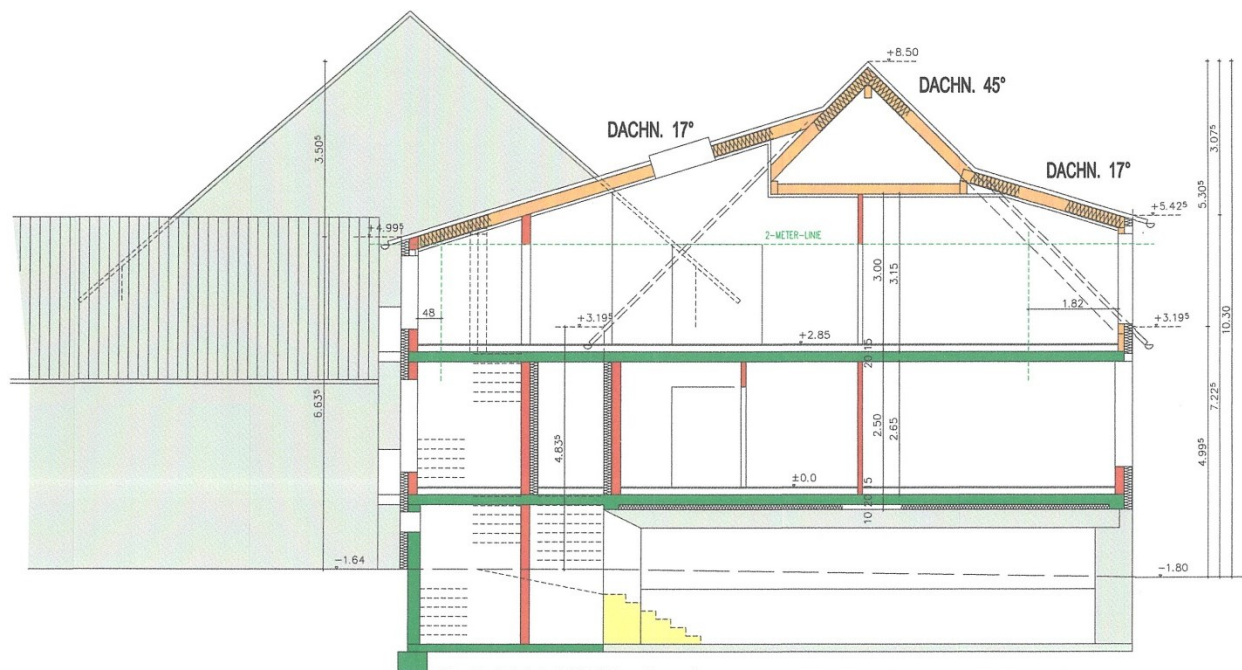
SCHNITT A-A
