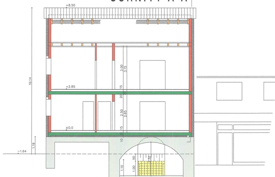
SCHNITT B-B
