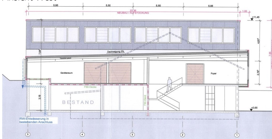
Ansicht Nord / Schnitt C-C
