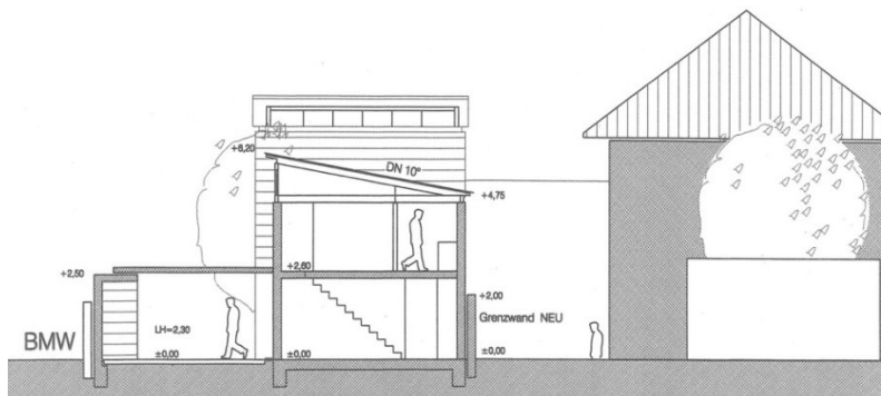
Schnitt Süd – Nord
