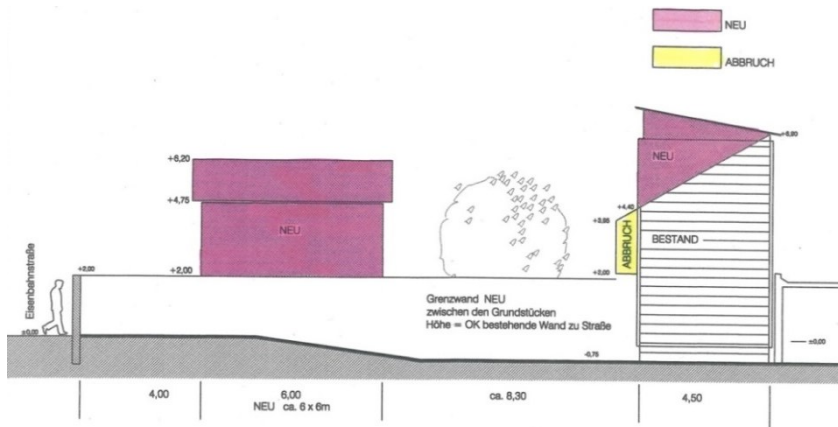
Ansicht Ost
