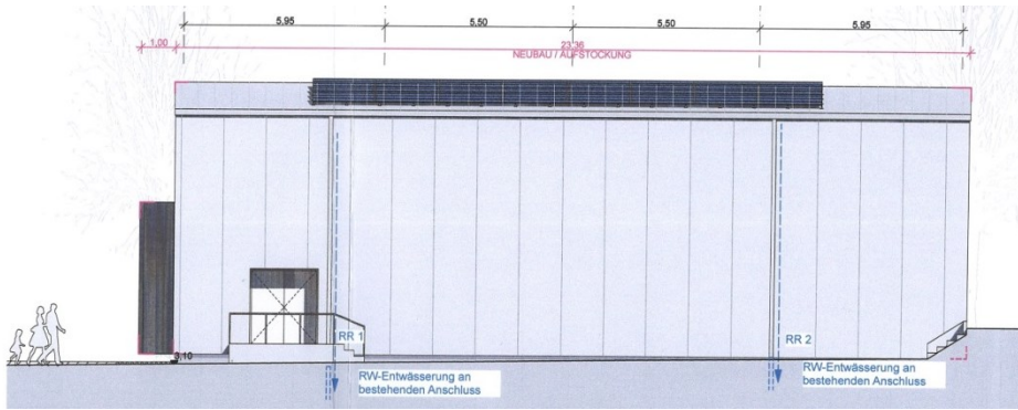
Ansicht Süd
