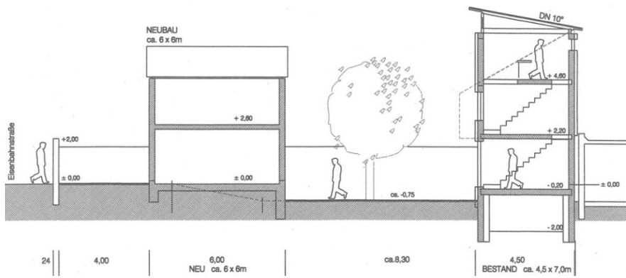
Schnitt Süd – Nord
