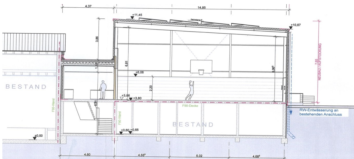
Schnitt B-B
