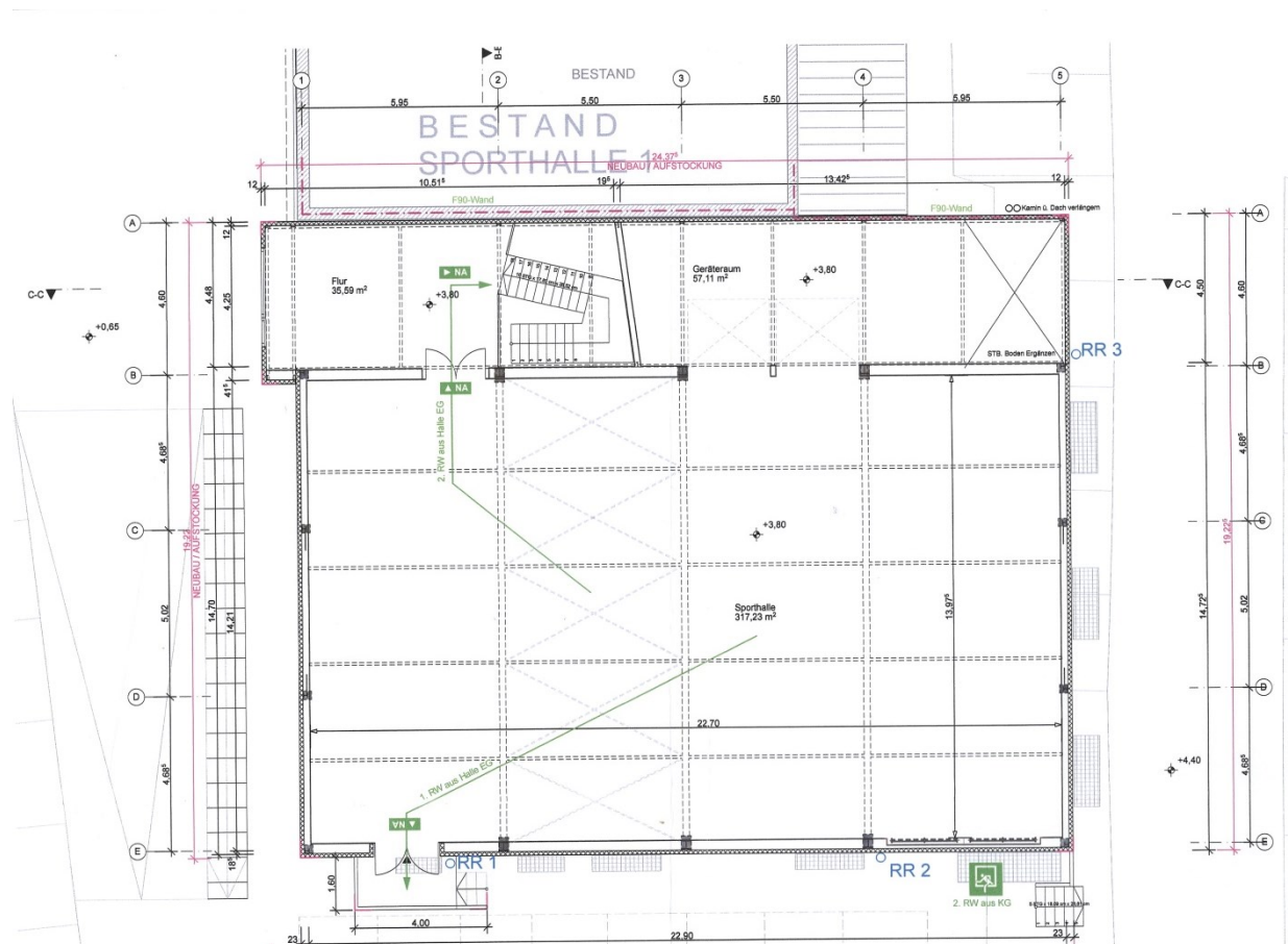
Grundriss EG
