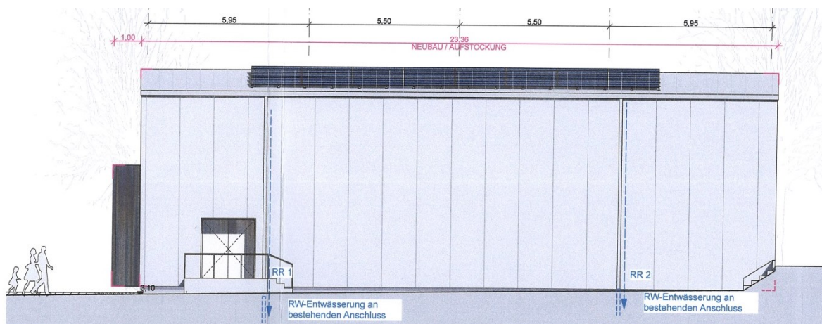
Ansicht Süd
