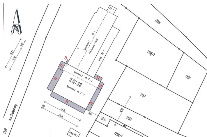
Abstandsflächen
