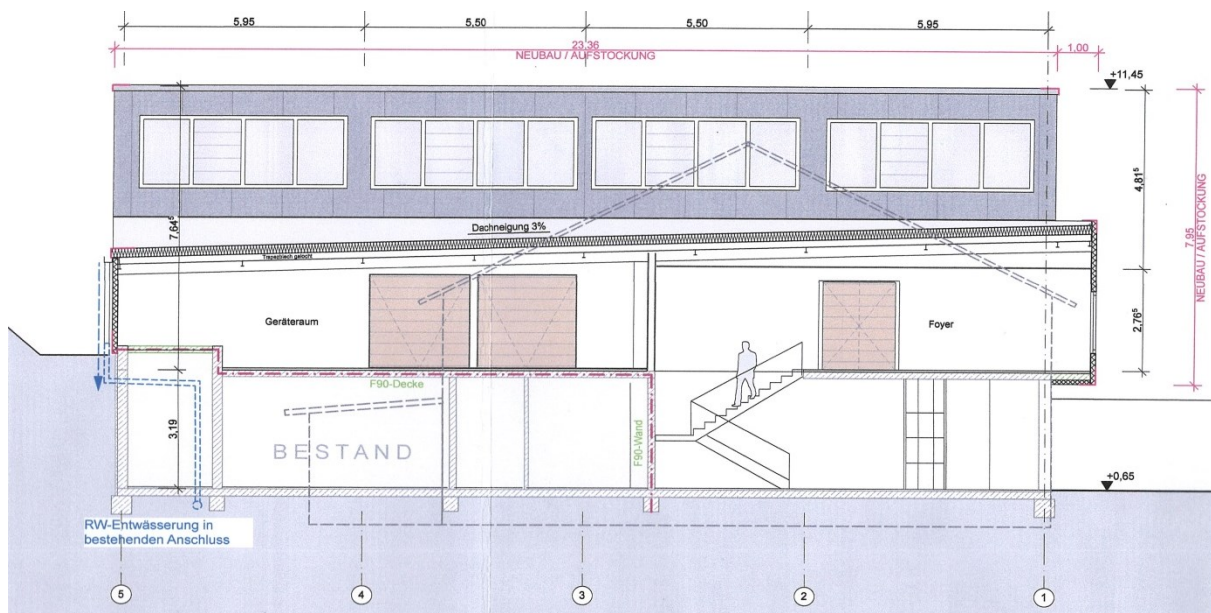
Ansicht Nord / Schnitt C-C
