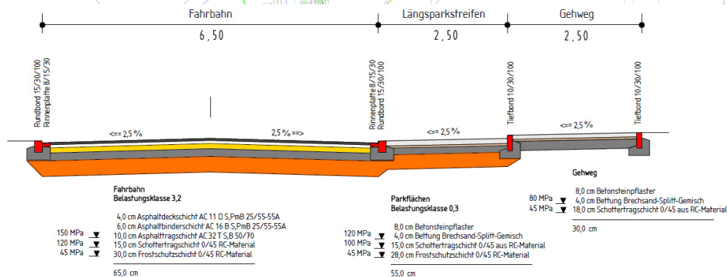
Querschnitt bei Station 0 + 125
